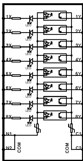
TYP DKS-35-11-xxx-x
